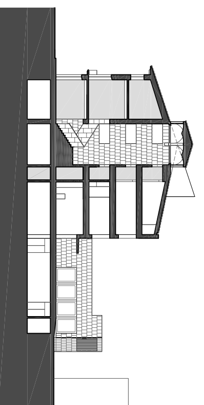
SECCIÓN LONGITUDINAL E 1/500
