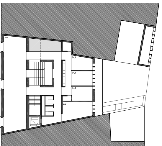
PLANTA PRIMERA E 1/500
