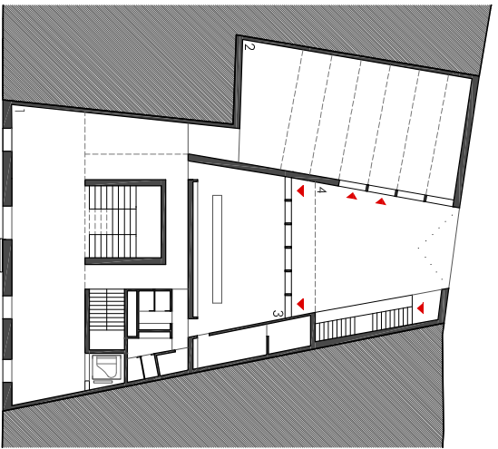
PLANTA BAJA E 1/500
