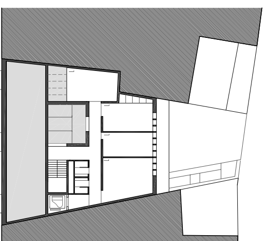
PLANTA ENTREPANTALLA E 1/500
